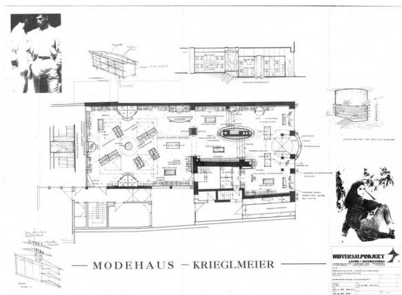
A Ladenplan Erdgeschoss (Bestandsunterlage)
